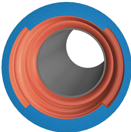
DN 300 till DN 500 monteras med fyra istället för två låselement, i motsvarande förankringsspår uppe och nere.
